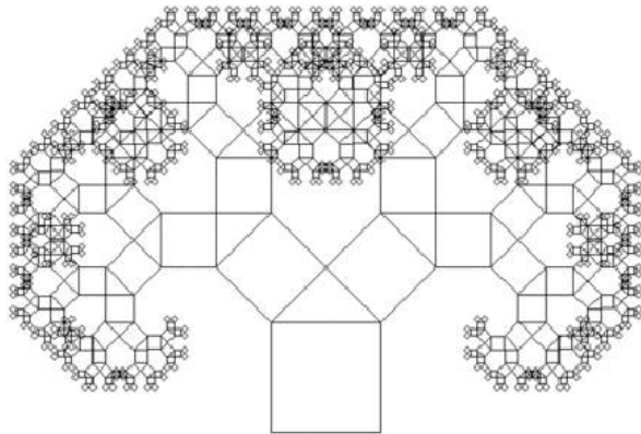
Мал. 2 Дерево Піфагора
